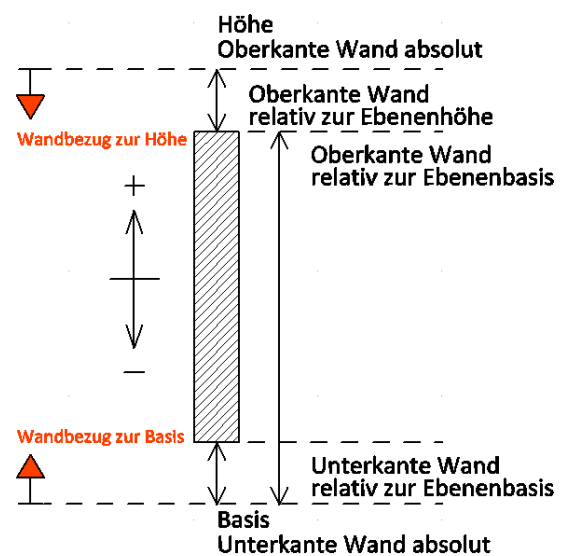
Abb.: Schema Wandparameter in SPIRIT und Bezug der Ebenenanpassung.
