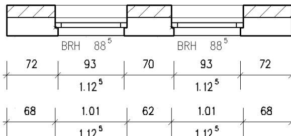
Abb.: Unterschied zwischen Anschlagbreite vermaßen: ja und nein in der Baugesuchs-Detaillierung.
